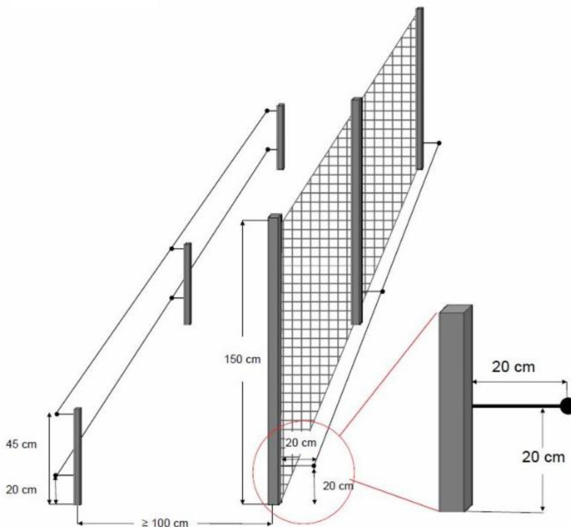
Slika 1: Primer postavitve dvojne ograje za plemenske svinje, tekače in pitance
